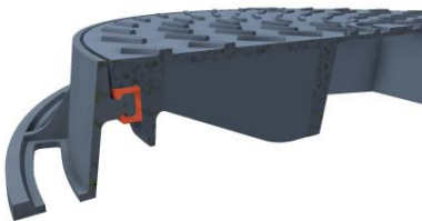
HYDROthen-csillapító betét
