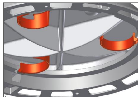
3-pontos rugókaros zárás
